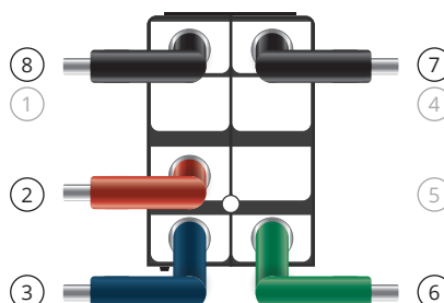
KABELBOOM (BACK)
